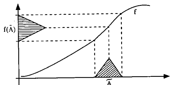
اصل گسترش برای یک تابع صعودی یک‌نواخت
