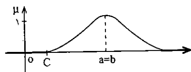
شکل ۱ نمونه‌ای از یک عدد فازی با تکیه‌گاه کران‌دار
